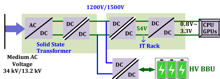
圖 1 未來 AI 伺服器系統之供電架構
